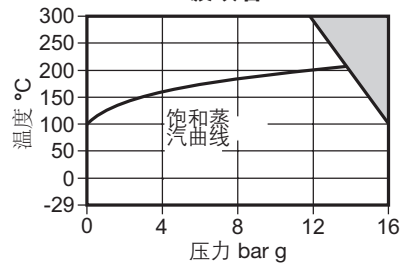
波纹管 B
