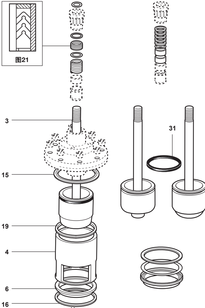
图22 平衡阀芯
